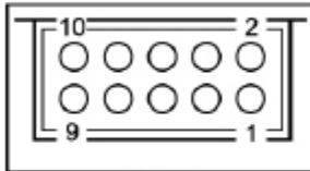
CN3
